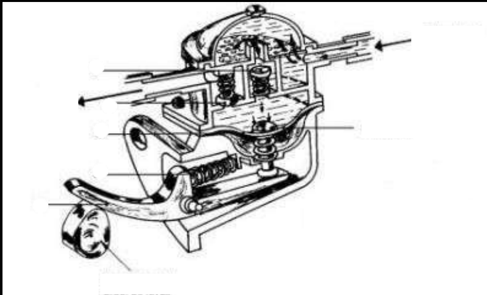
Figura 4. Bomba de alimentación de membrana
