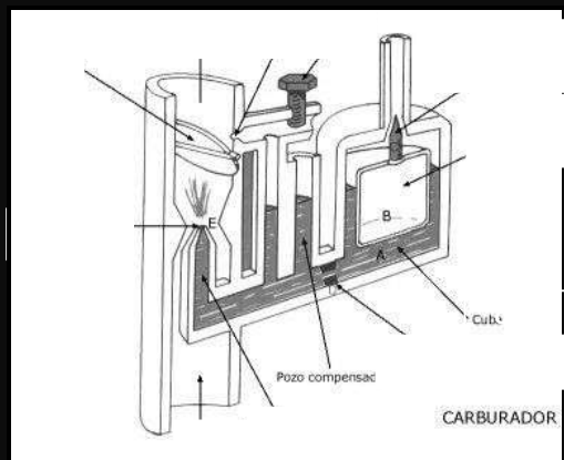
Figura 5. Carburador
